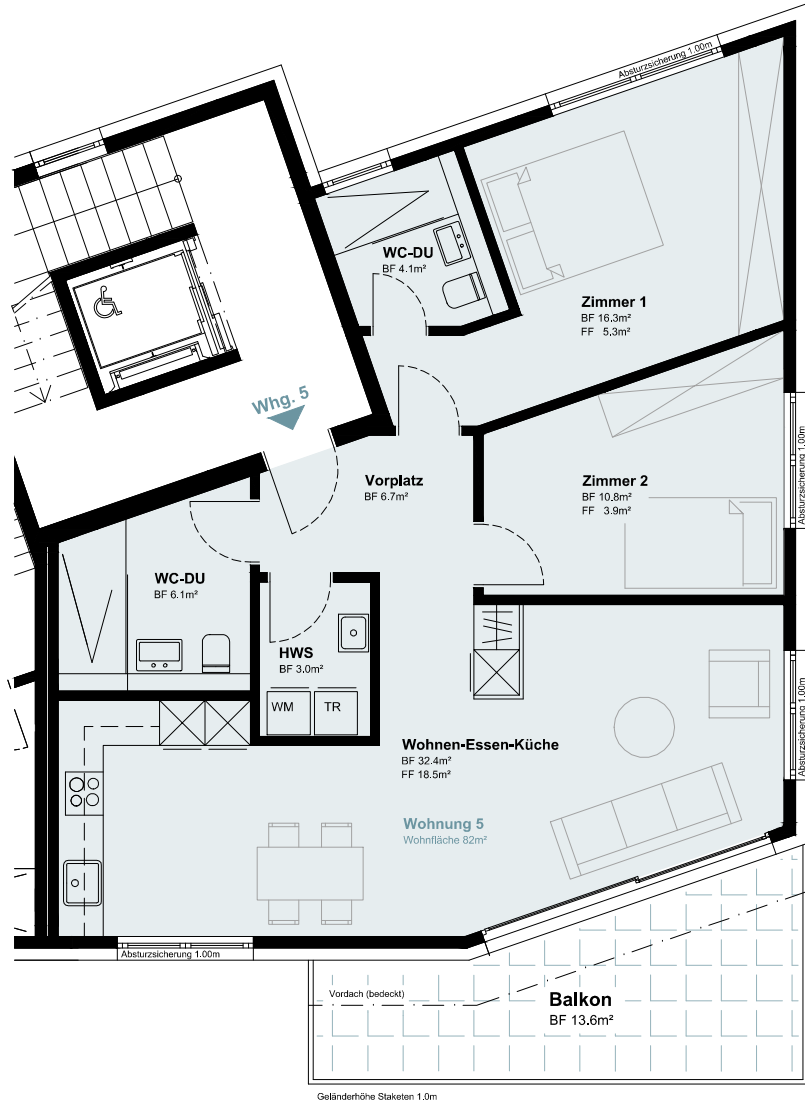
Wohnungsgrundriss / WHG 5 - 3. OG (Mst. 1:100)
