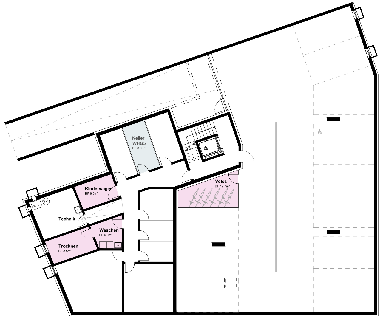
Grundriss Untergeschoss (massstablos)
