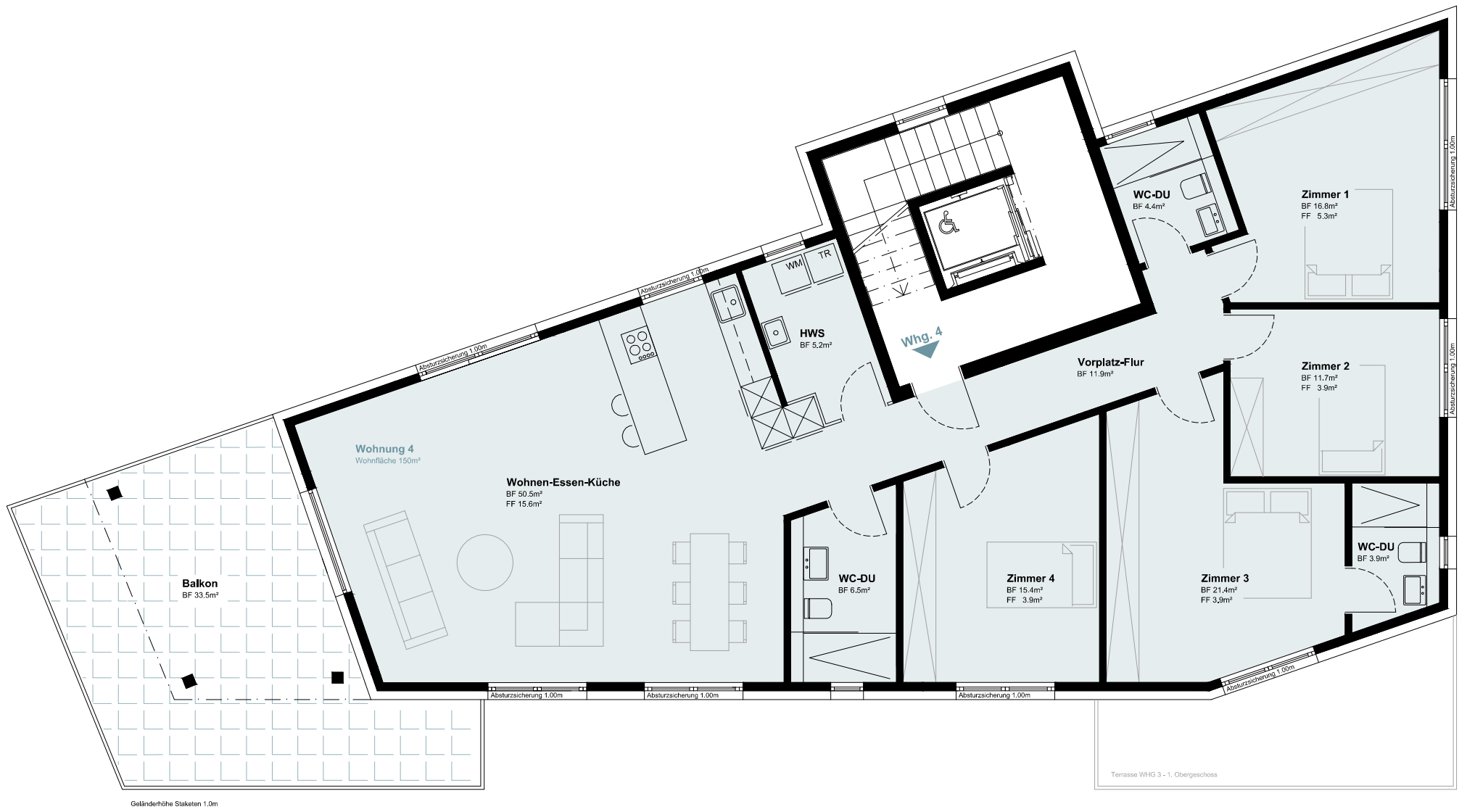
Wohnungsgrundriss / WHG 4 - 2. OG (Mst. 1:100)
