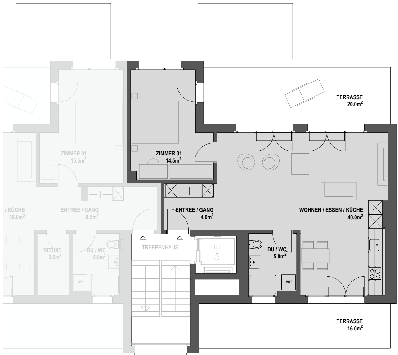
Grundriss Mst 1:100
