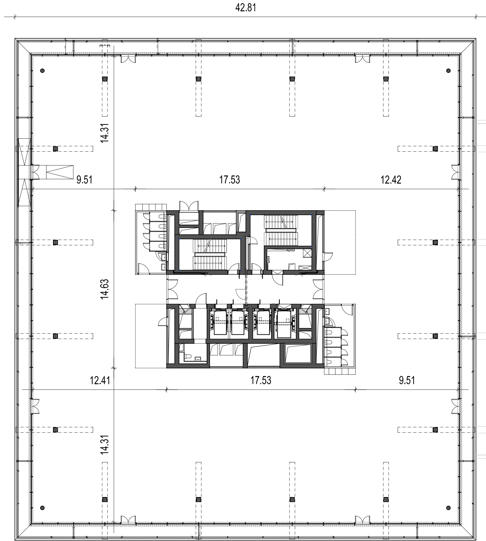
ALBA Haus Grundriss Regelgeschoss
