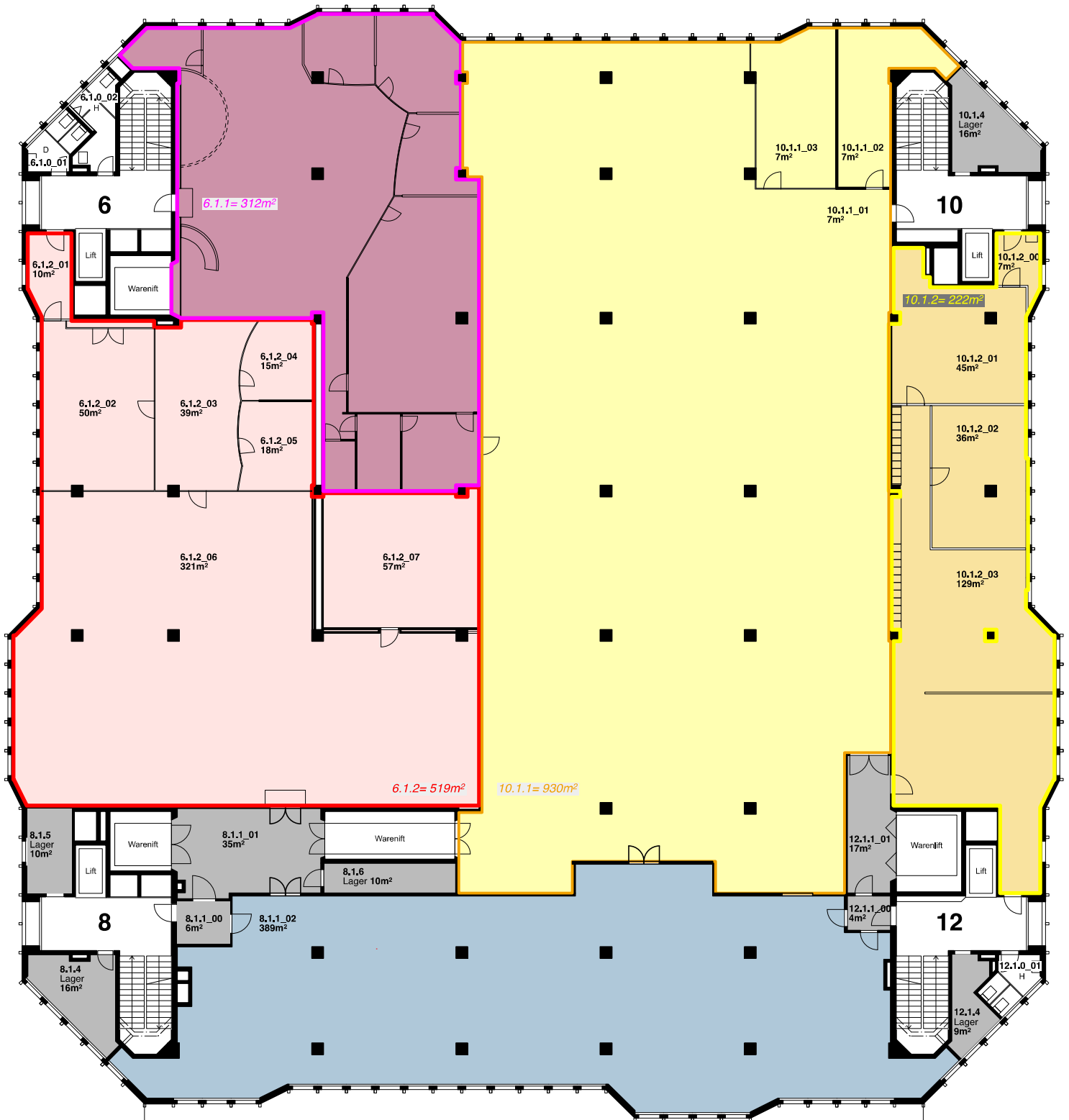
004 1.OG Ganzes Haus A3 1/200
