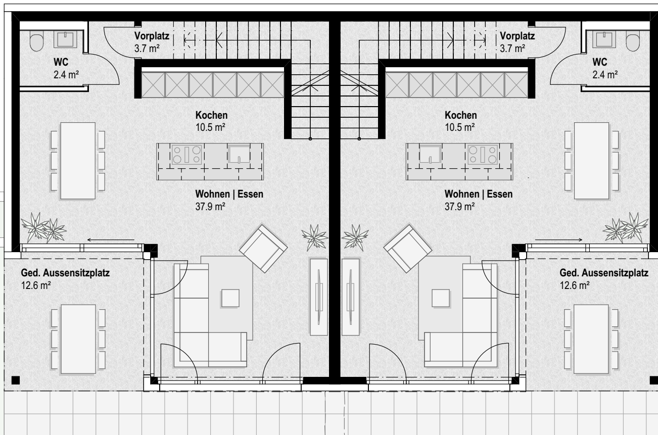
Erdgeschoss Doppel - EFH
