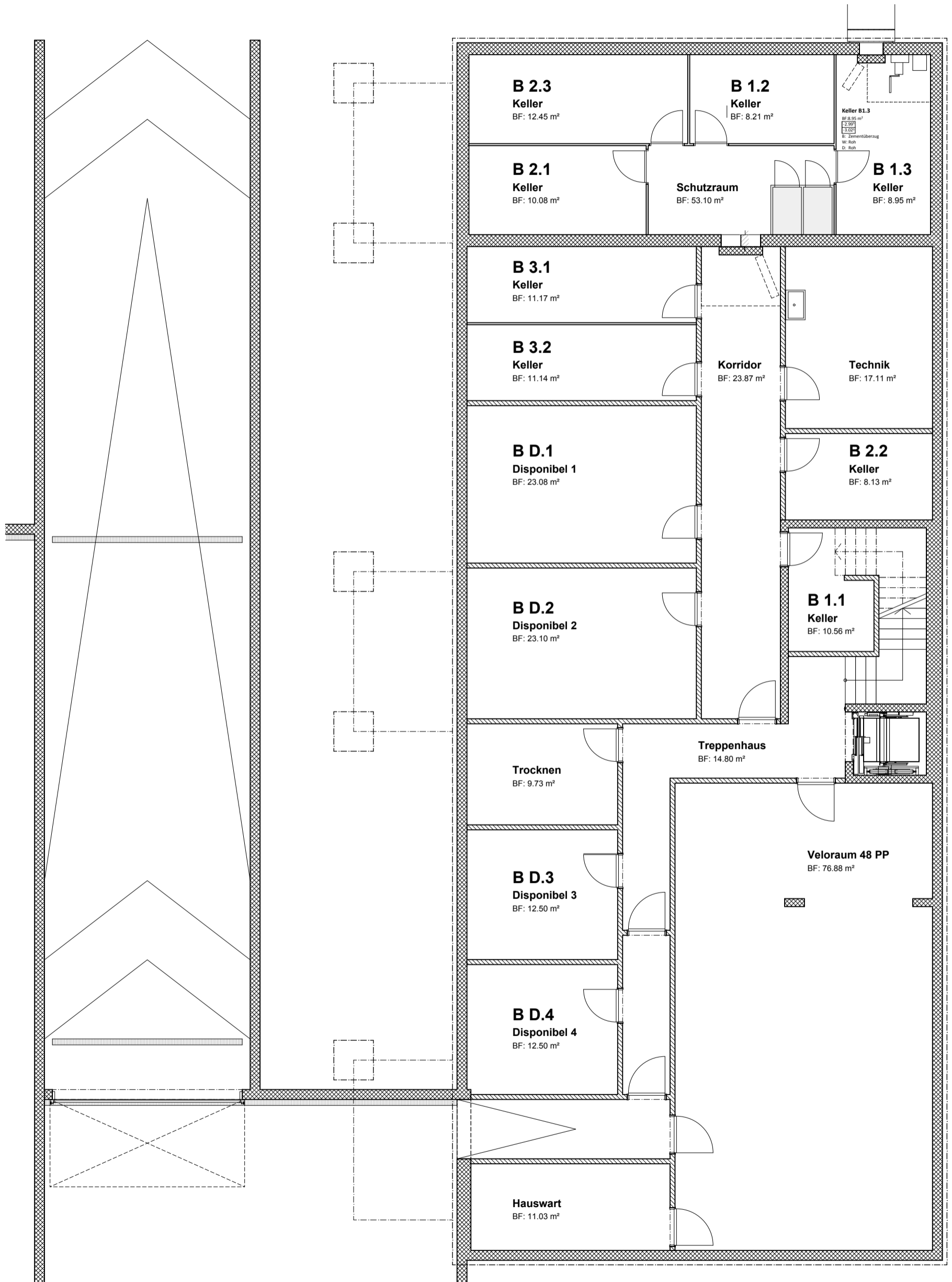
HAUS B | Untergeschoss
