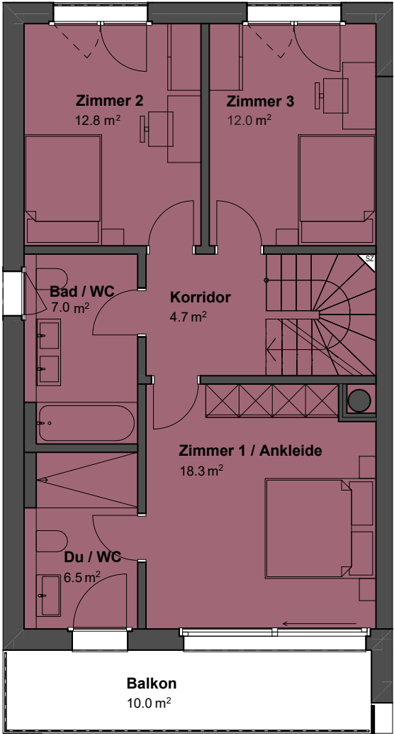
Obergeschoss 69.2 m²
