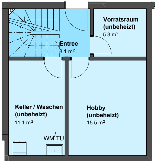
Untergeschoss 41.9 m²
