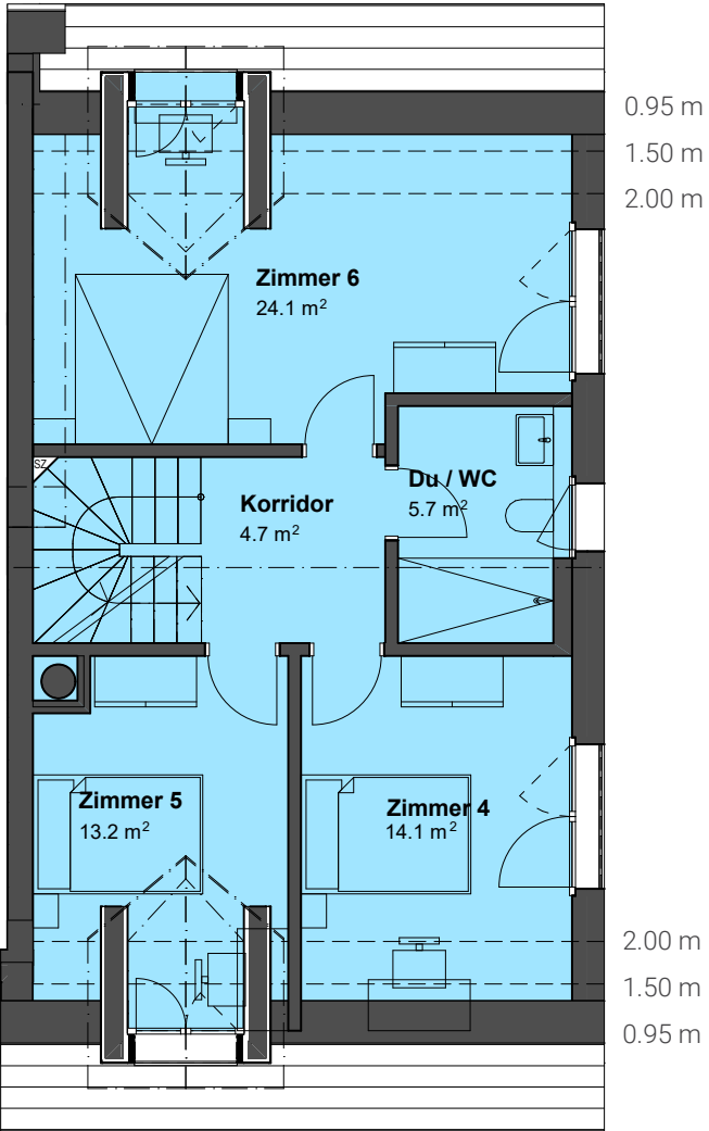
1. Dachgeschoss 69.2 m²
