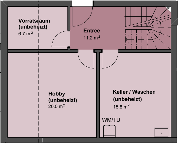
Untergeschoss 56.1 m²
