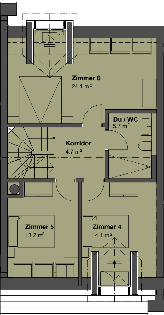
1. Dachgeschoss 69.2 m²
