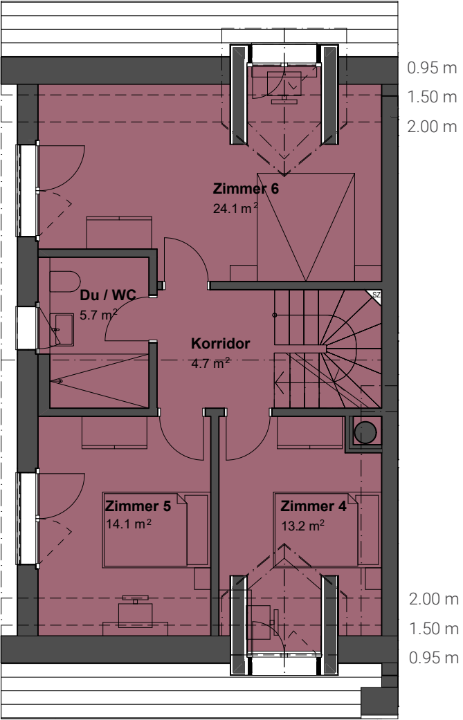
1. Dachgeschoss 69.2 m²
