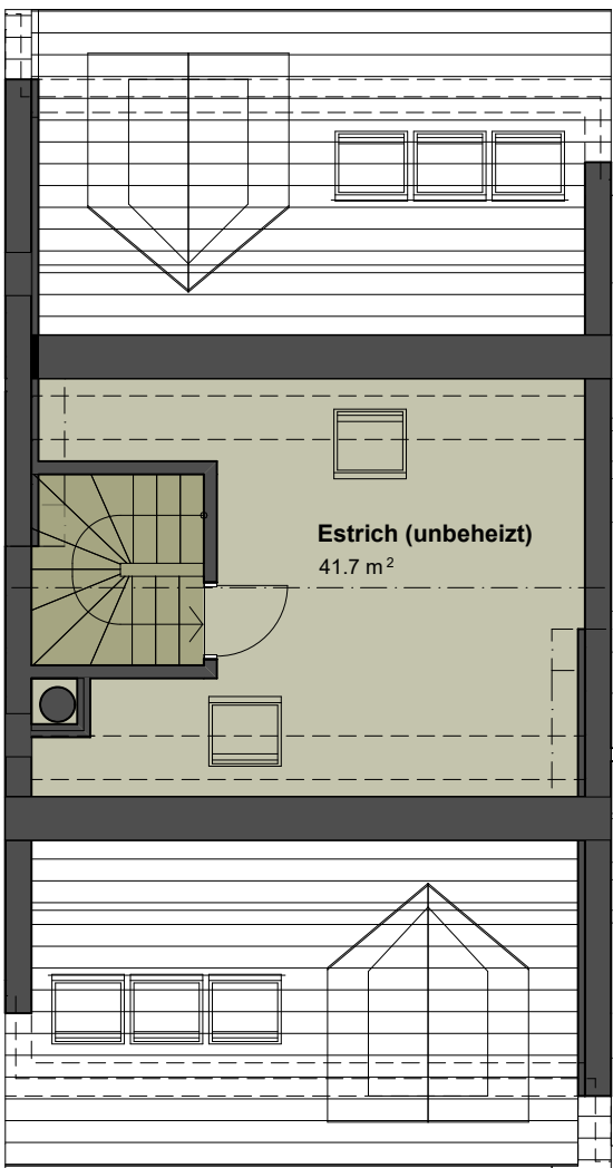
2. Dachgeschoss 47.0 m²
