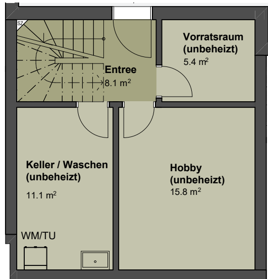
Untergeschoss 42.3 m²
