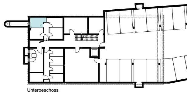
Untergeschoss
