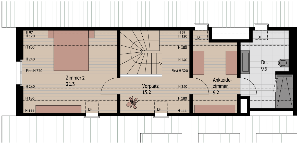
2. Dachgeschoss
