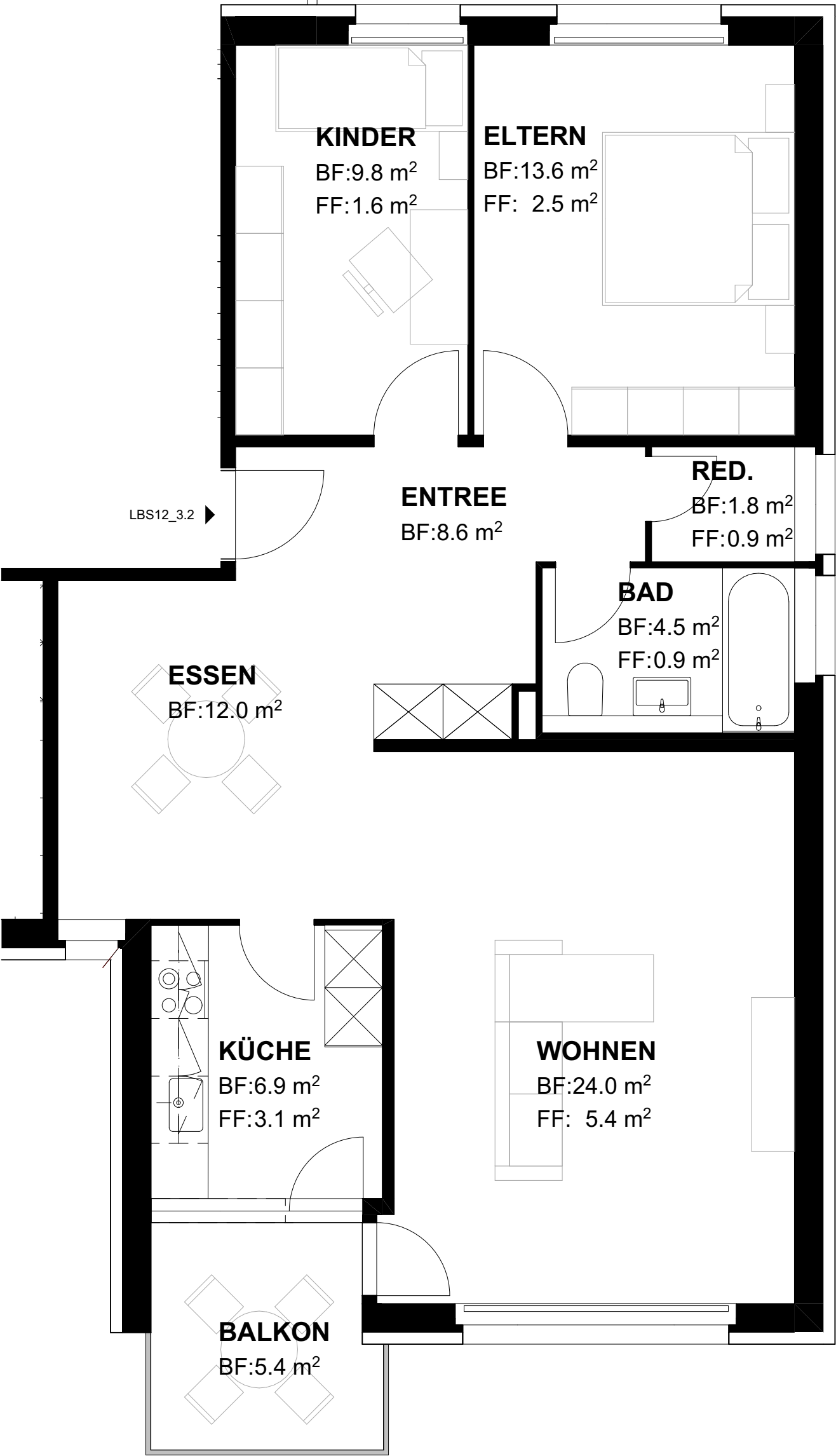
WOHNUNG LBS12_3.2
