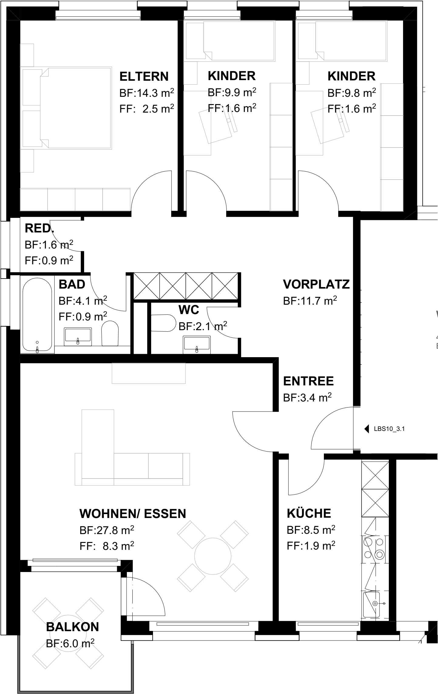
WOHNUNG LBS10_3.1
