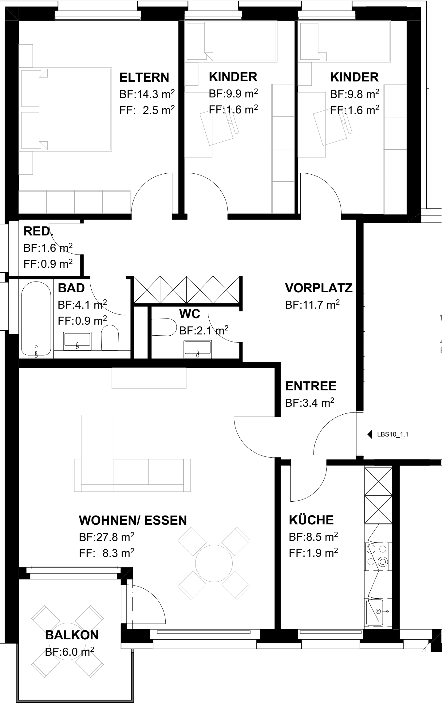
WOHNUNG LBS10_1.1
