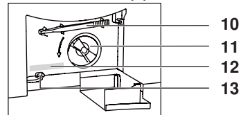
Ablaufbehälter (4)
