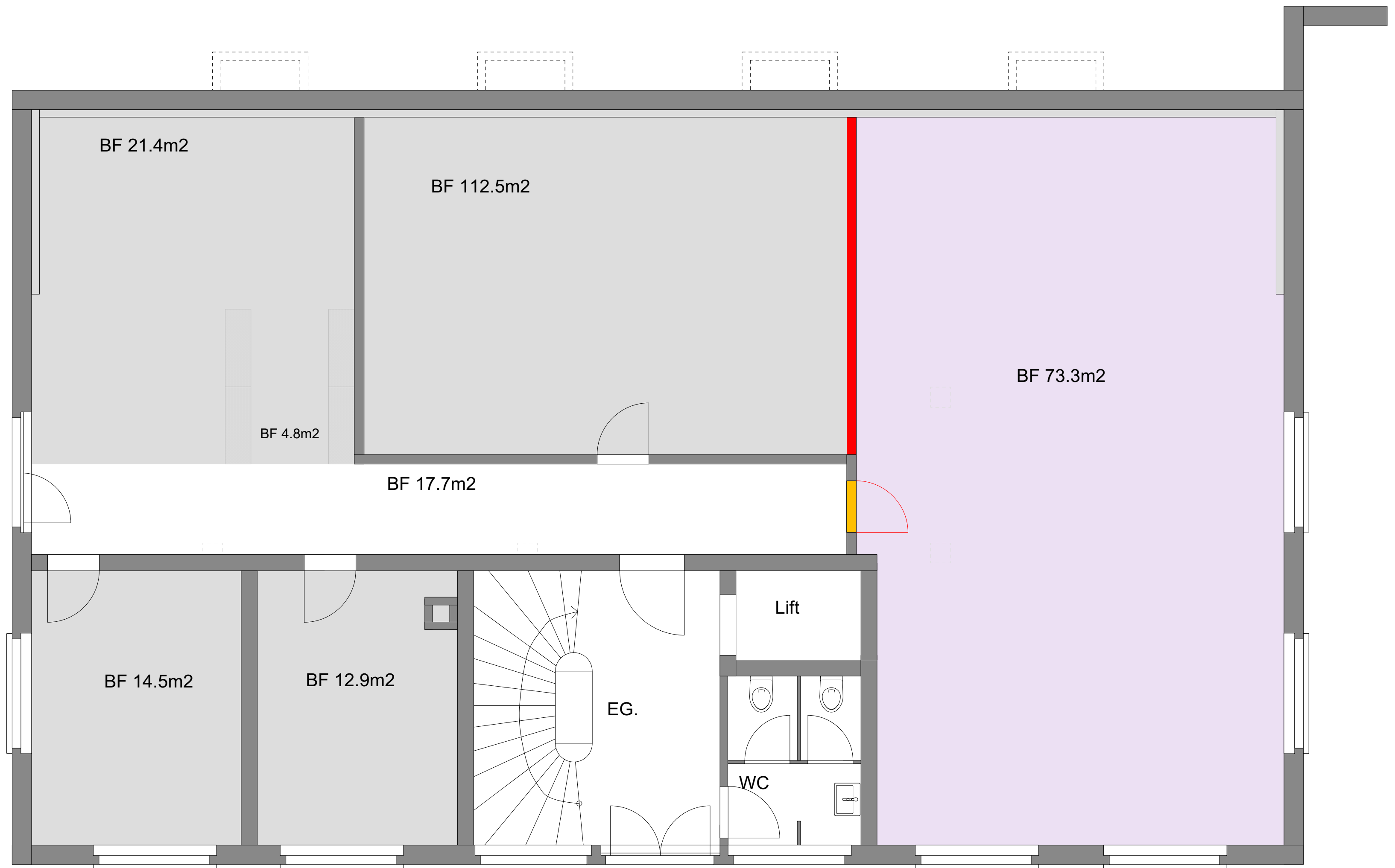
Erdgeschoss, Lager / Werkstatt
