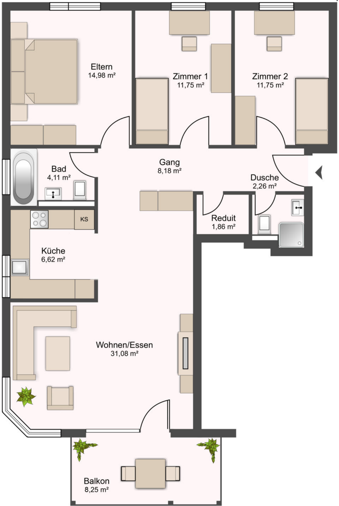
4.5 Zimmer - 1. OG - Ca. 93 m 2 - Südstrasse 2 - Nr. 2400.02.4130
