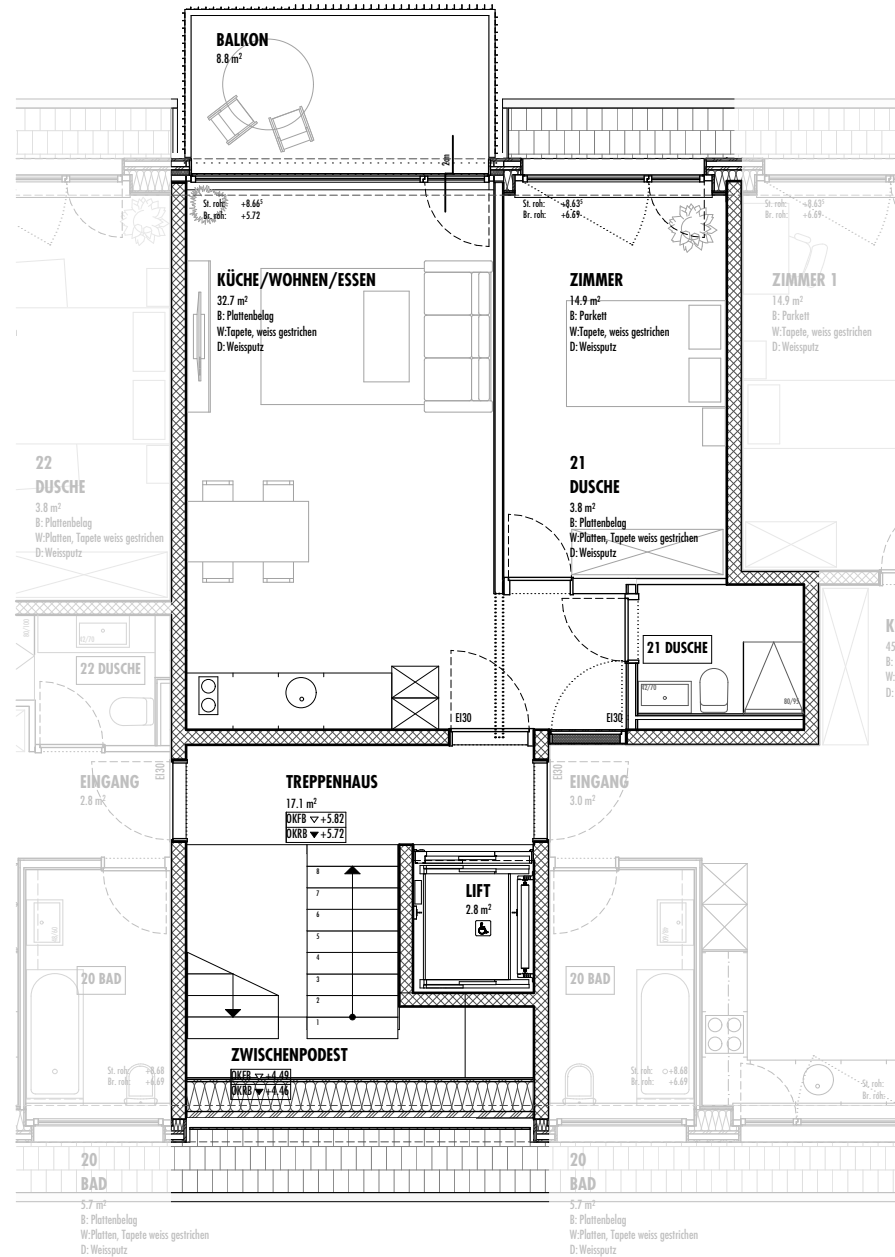
GRUNDRISS DG - 1:100
