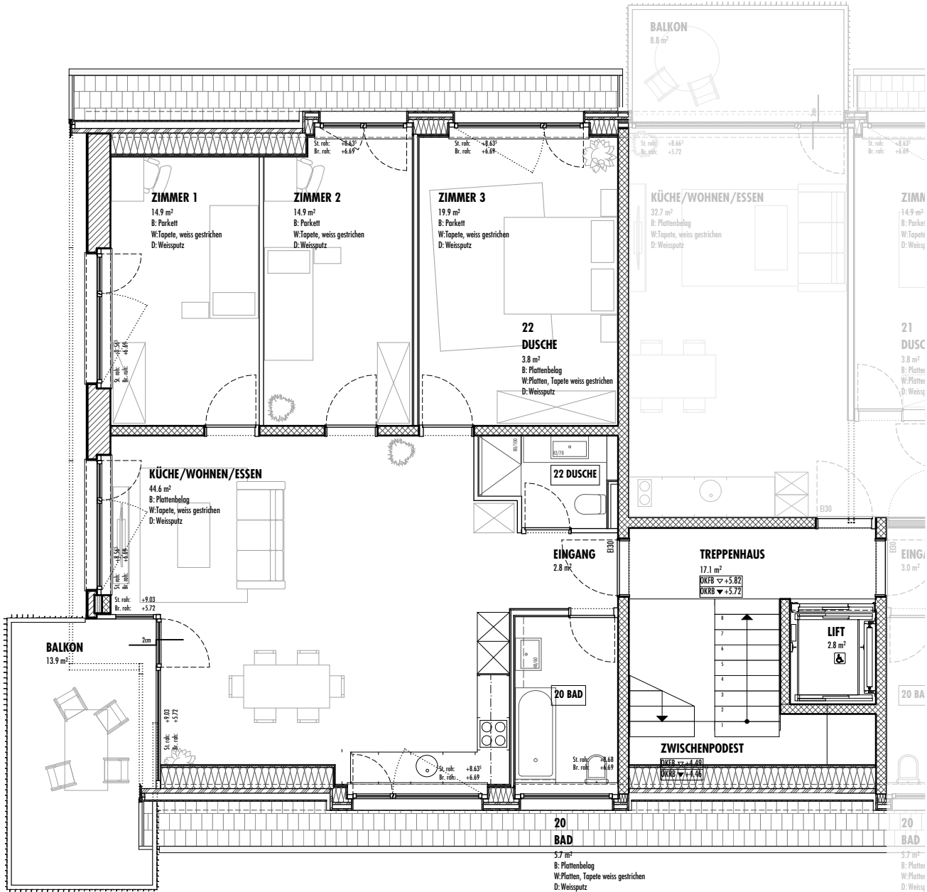
GRUNDRISS DG - 1:100
