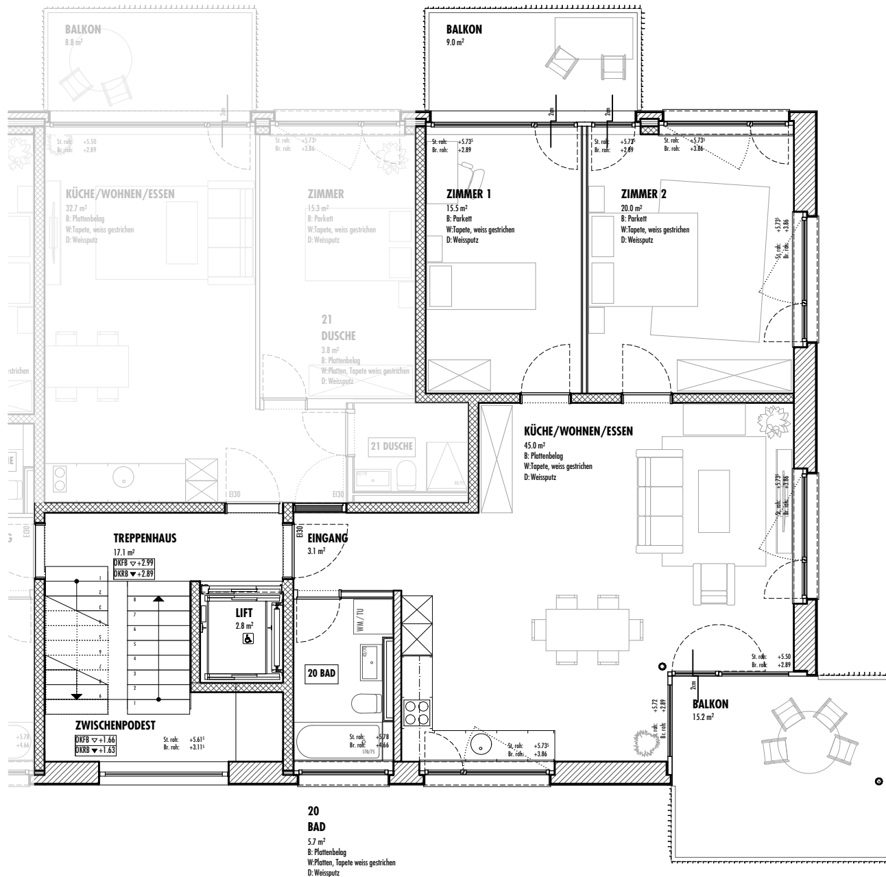
GRUNDRISS OG - 1:100
