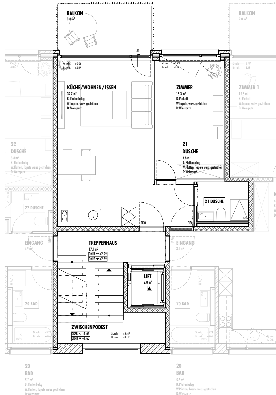
GRUNDRISS OG - 1:100
