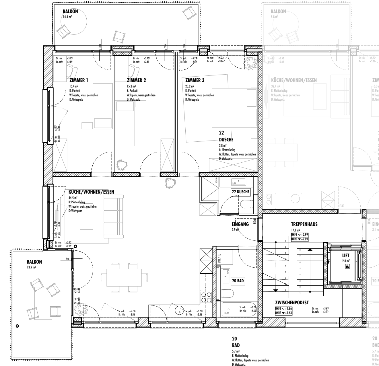
GRUNDRISS OG - 1:100
