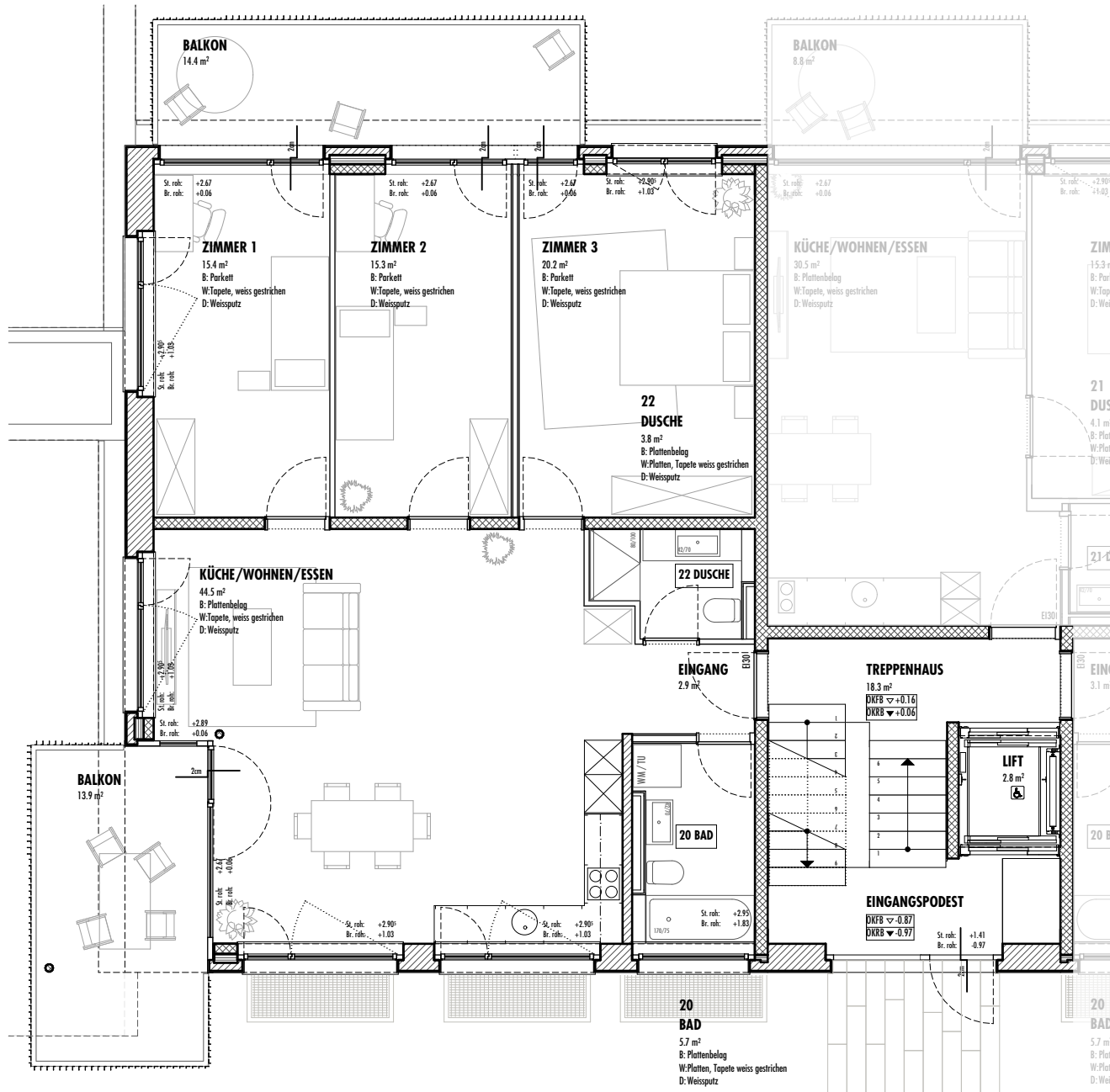
GRUNDRISS EG - 1:100
