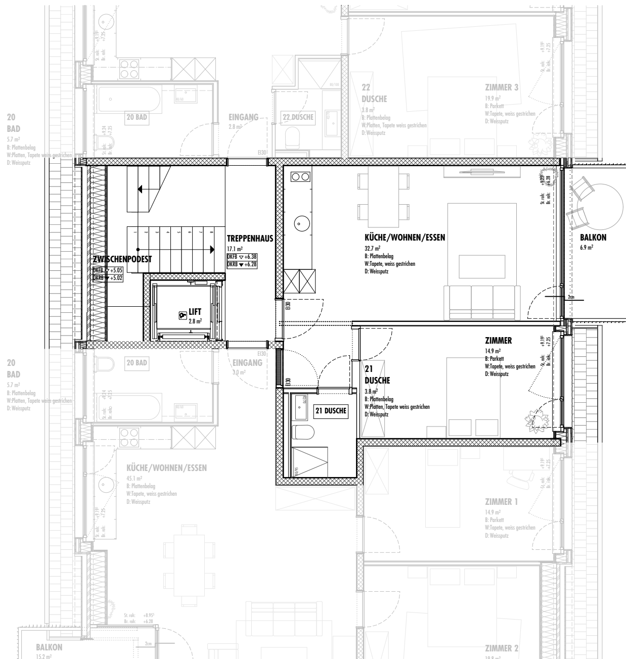
GRUNDRISS DG - 1:100
