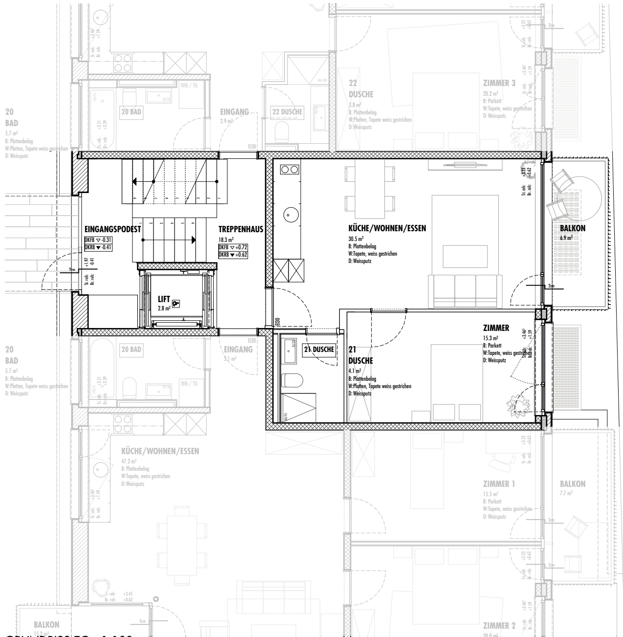
GRUNDRISS EG - 1:100
