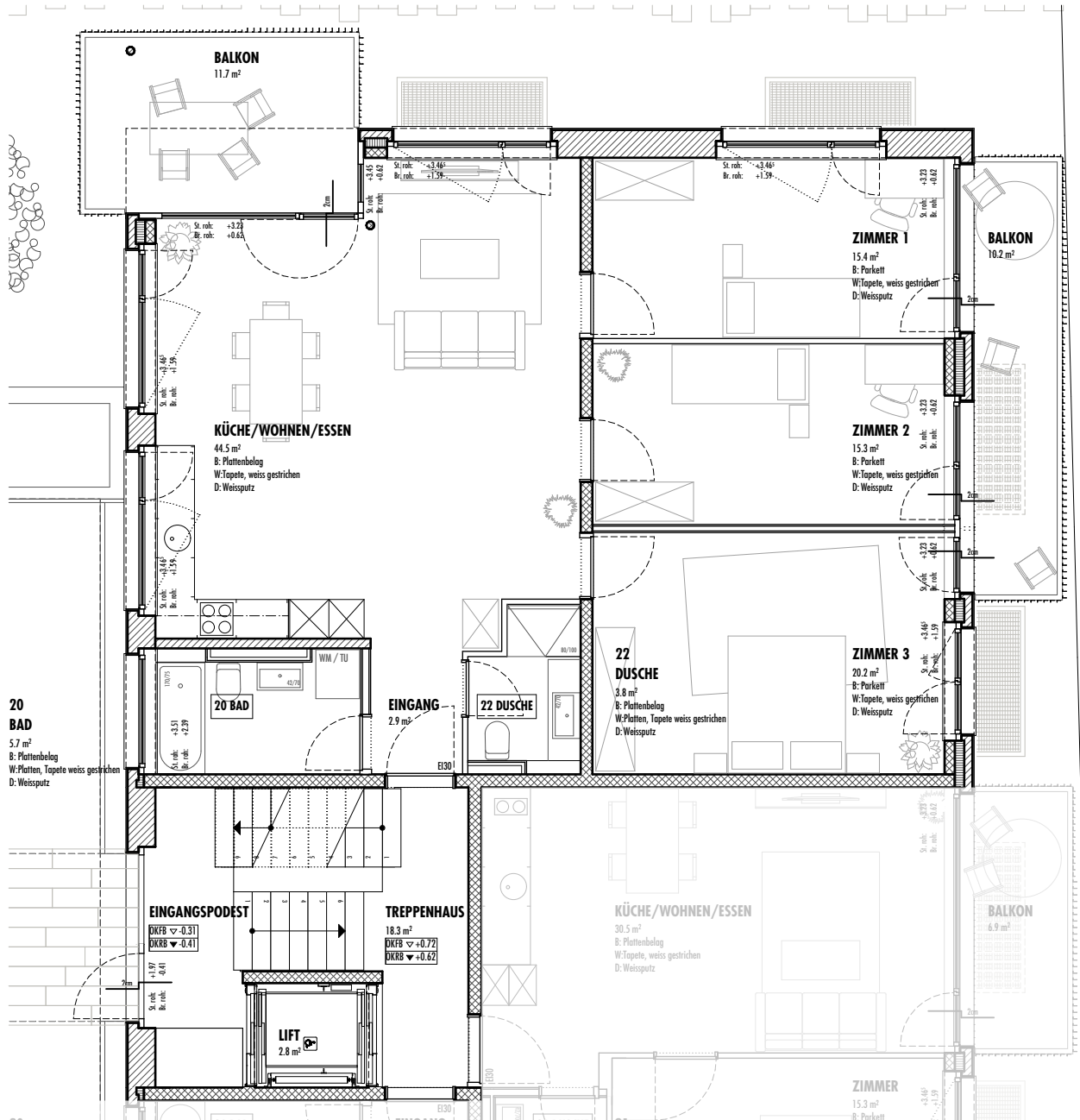
GRUNDRISS EG - 1:100
