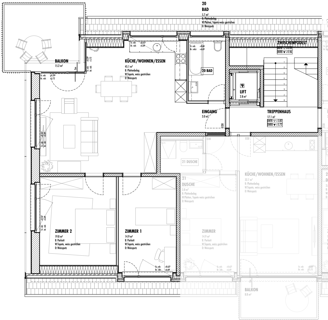
GRUNDRISS DG - 1:100
