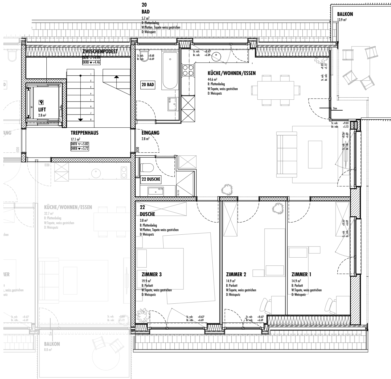
GRUNDRISS DG - 1:100
