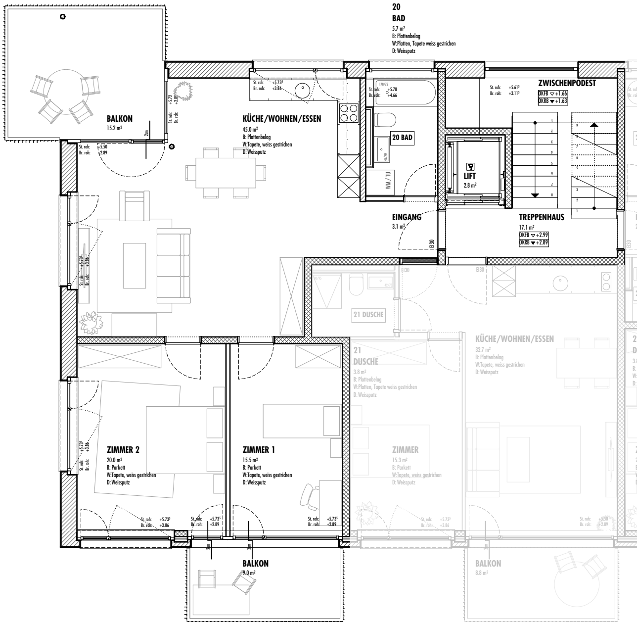
GRUNDRISS OG - 1:100
