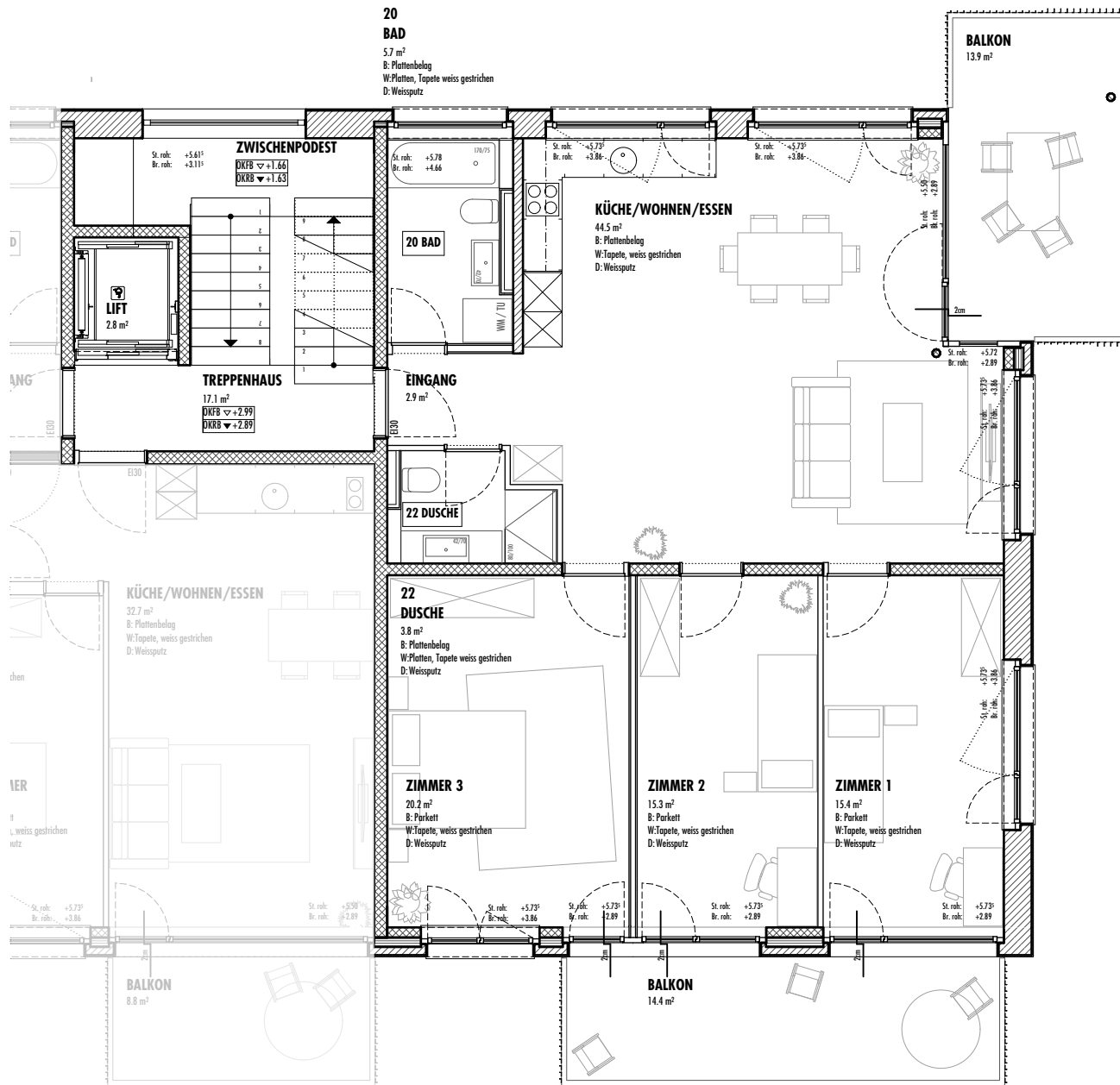
GRUNDRISS OG - 1:100
