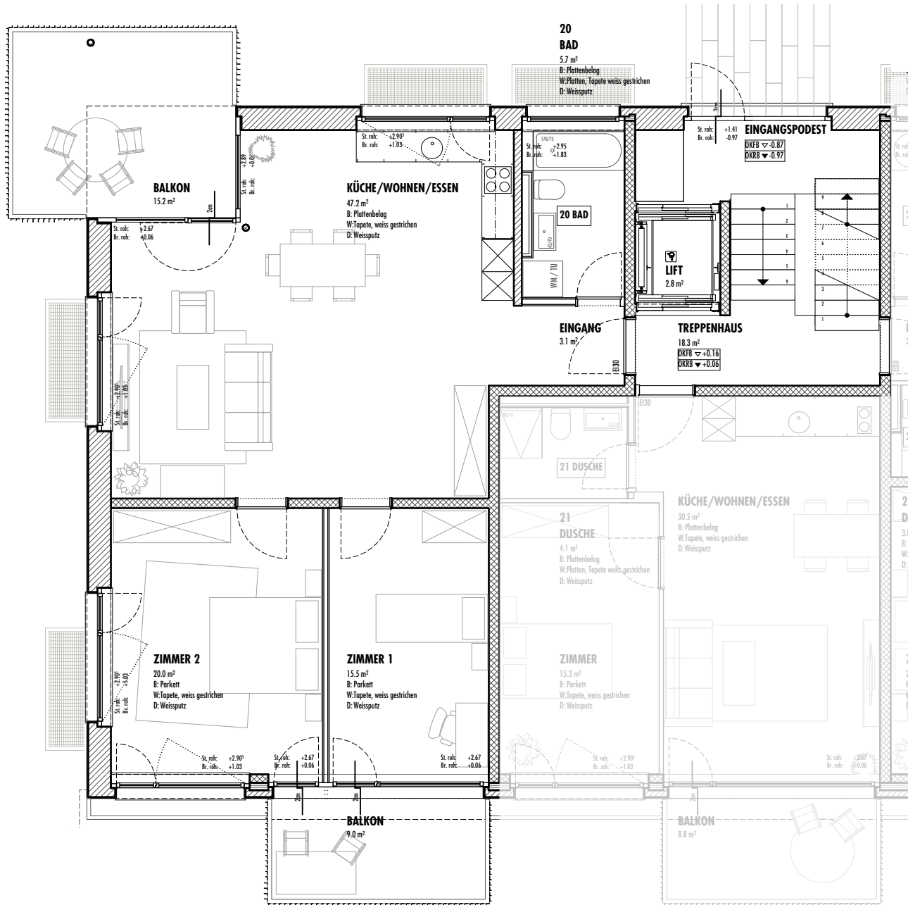
GRUNDRISS EG - 1:100
