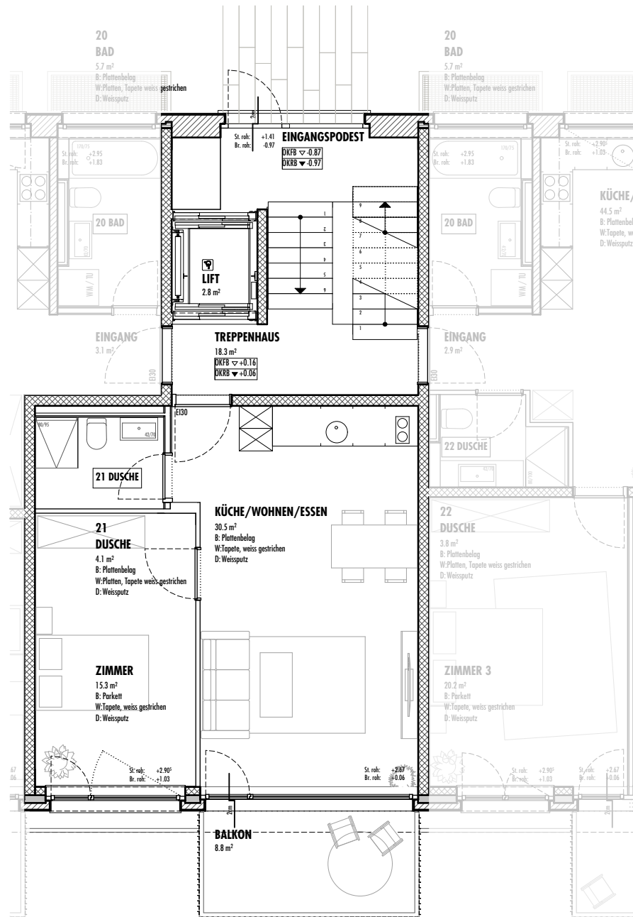
GRUNDRISS EG - 1:100
