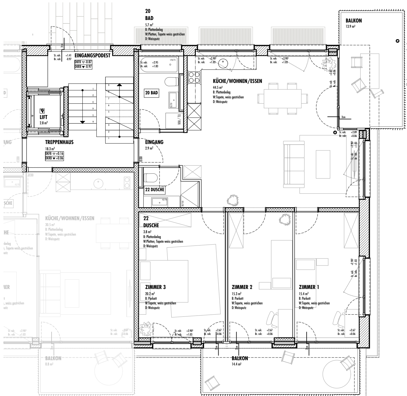
GRUNDRISS EG - 1:100
