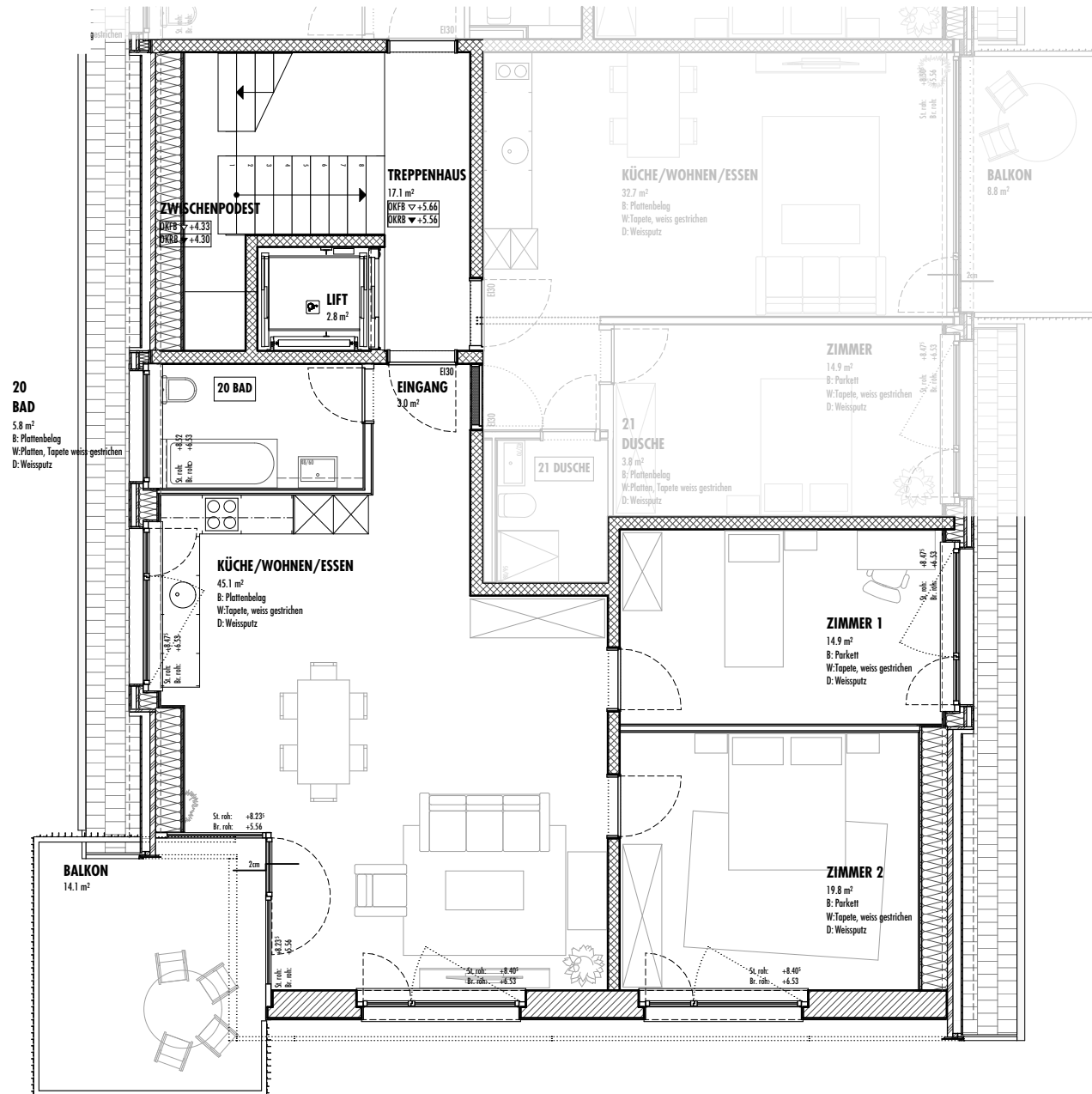
GRUNDRISS DG - 1:100
