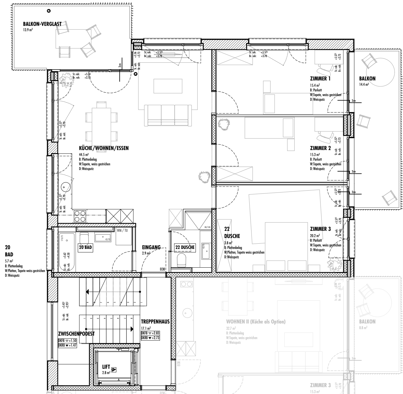
GRUNDRISS OG - 1:100
