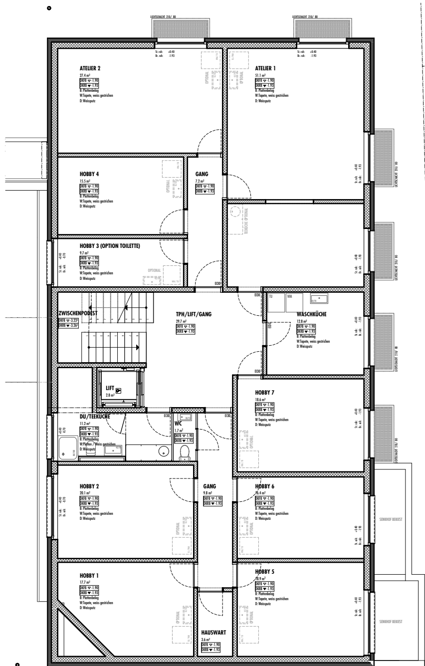
GRUNDRISS SG - 1:150
