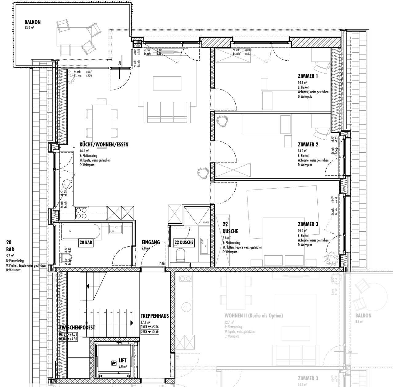
GRUNDRISS DG - 1:100
