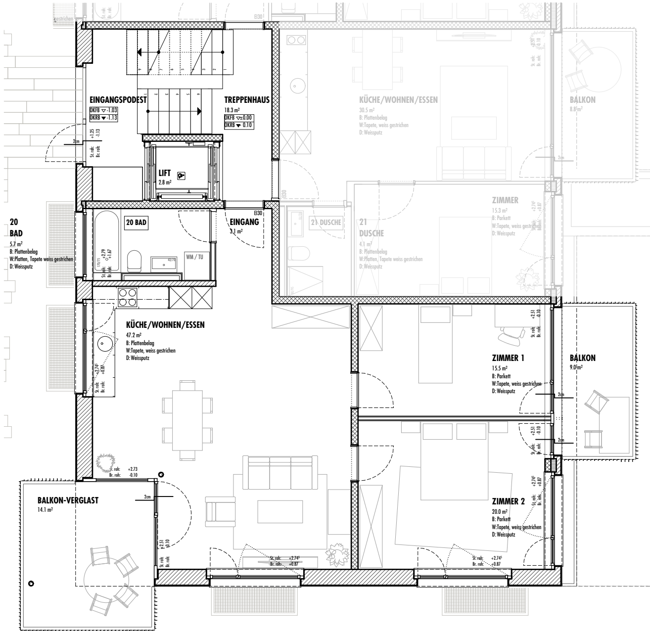
GRUNDRISS EG - 1:100
