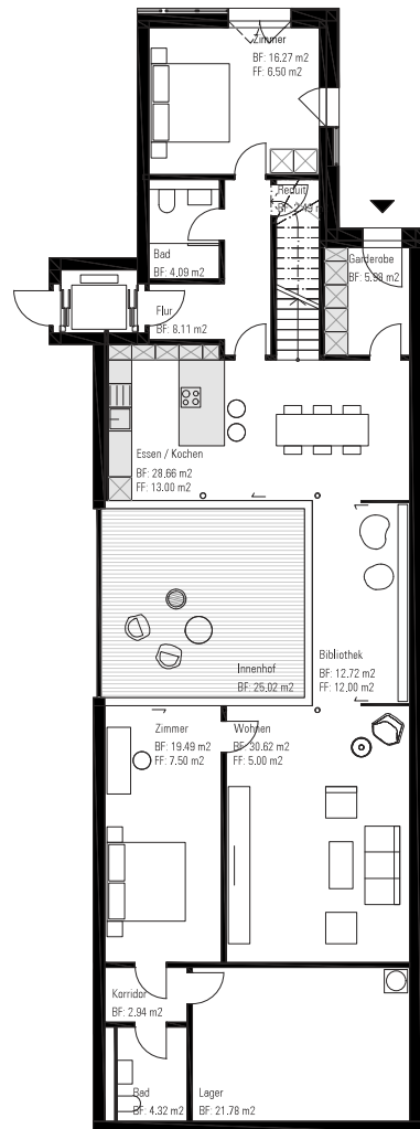
Erdgeschoss
