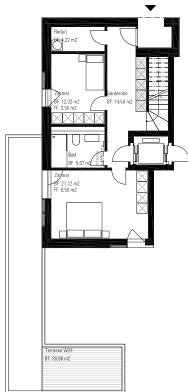
1.Obergeschoss
