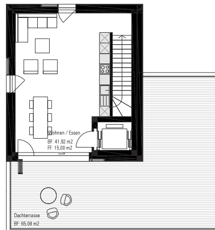
2.Obergeschoss
