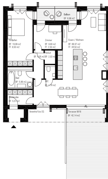
1. Obergeschoss
