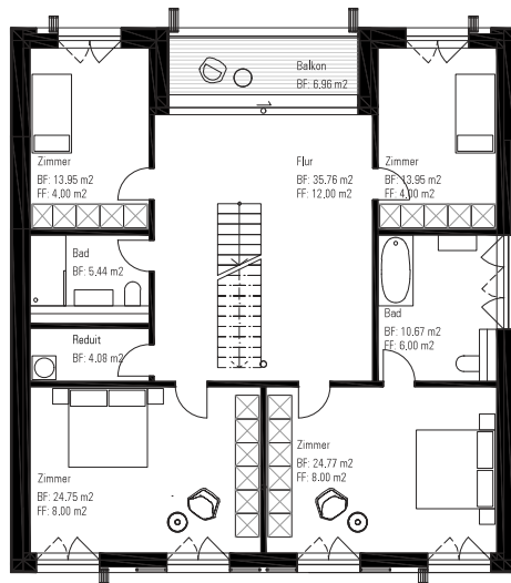
2.Obergeschoss
