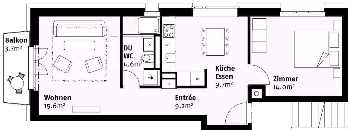
Wohnung 06.200 2.5 Zi-Whg. BF 53.1m 2
