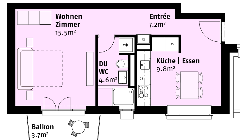
Wohnung 06.100 1.5 Zi-Whg. BF 37.1m 2
