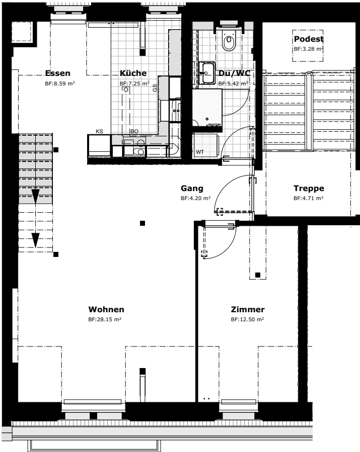
5.Obergeschoss
