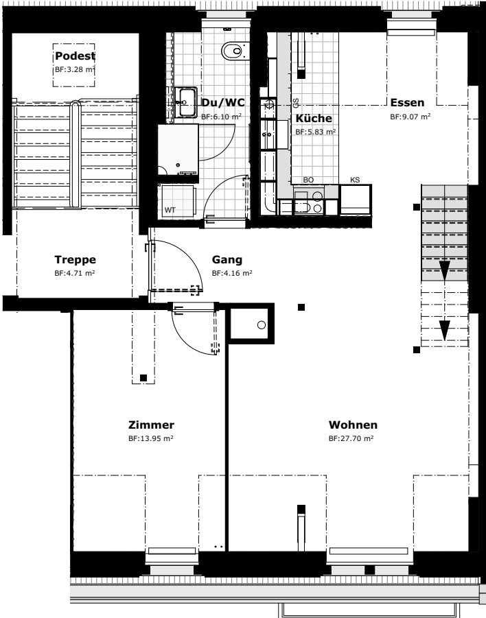
5.Obergeschoss
