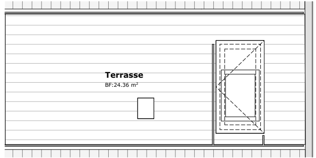
Dachaufsicht
