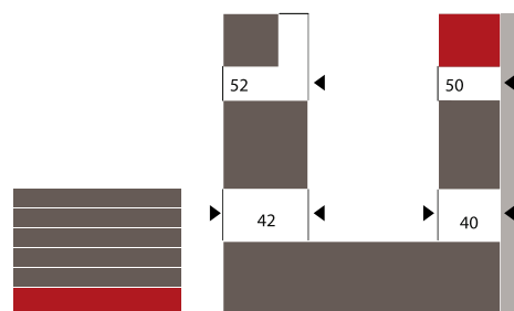
Ansicht Grundriss
