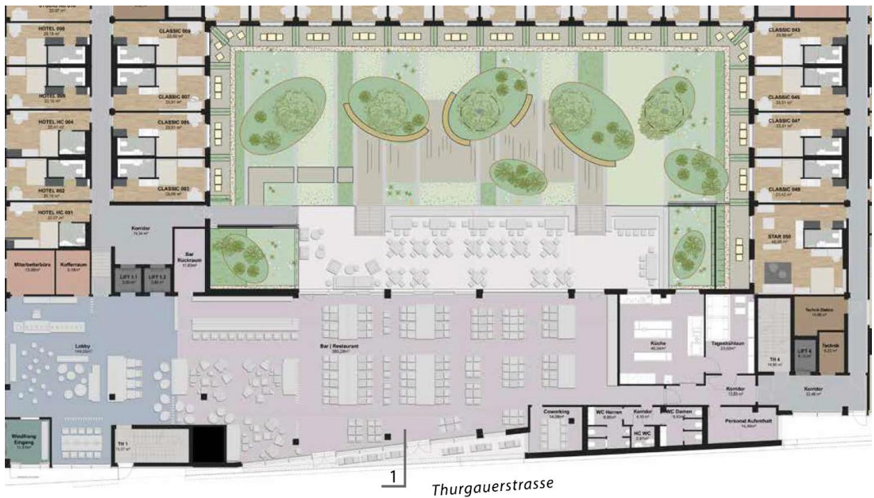
Grundrissplan EG
