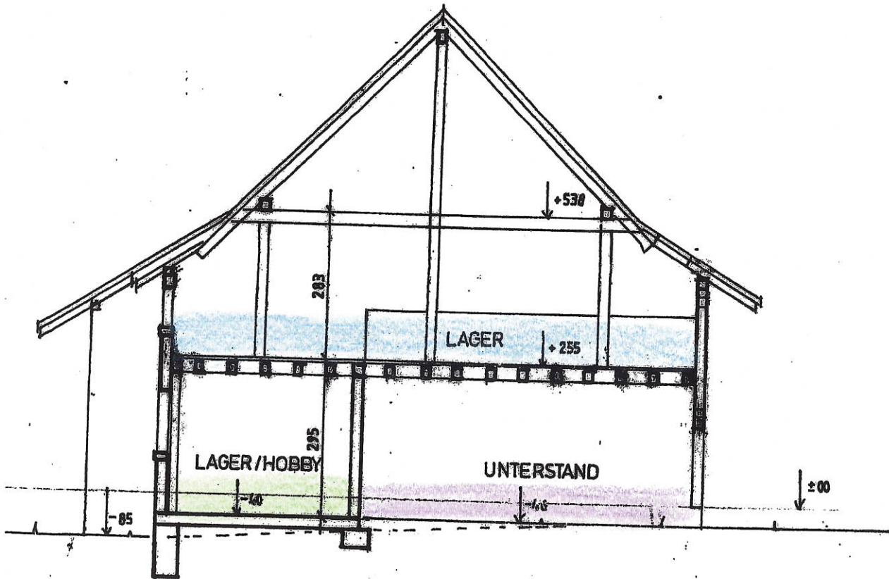
SCHNITT A—A
