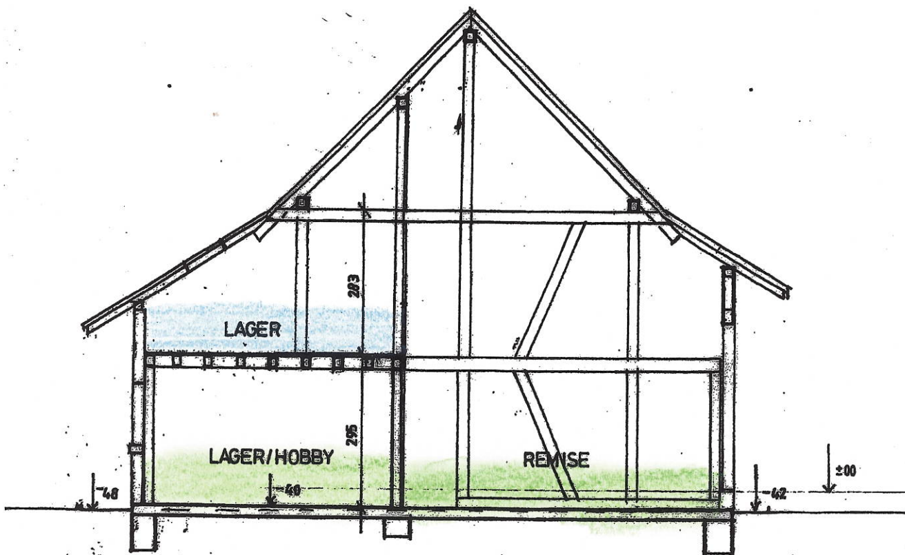
SCHNITT B—B
