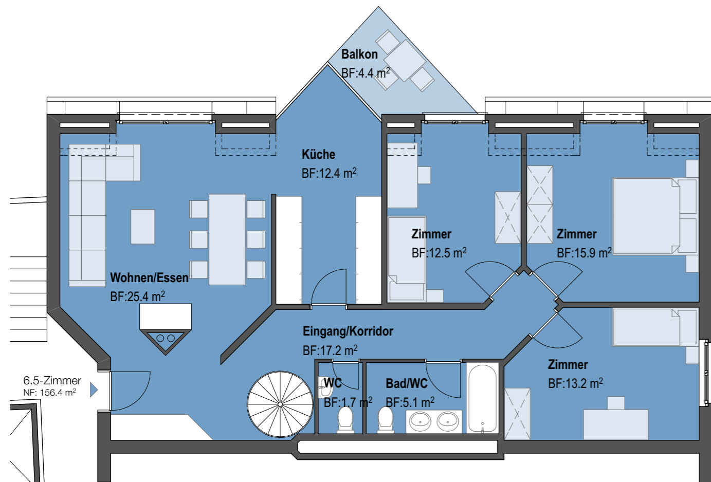
4. Obergeschoss
