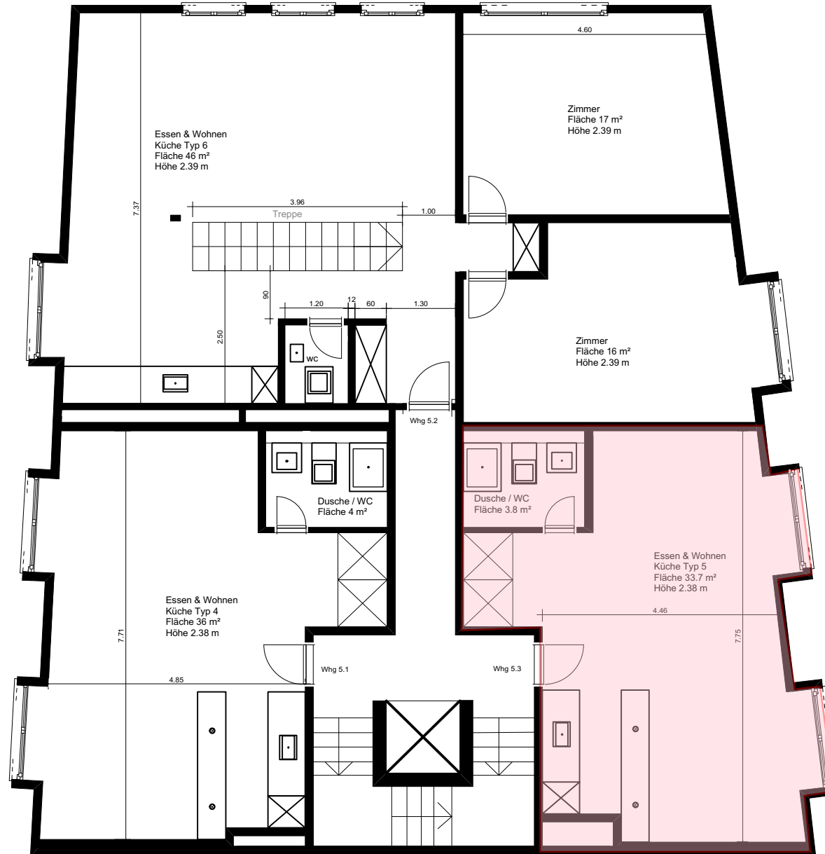
Grundriss 5.OG
