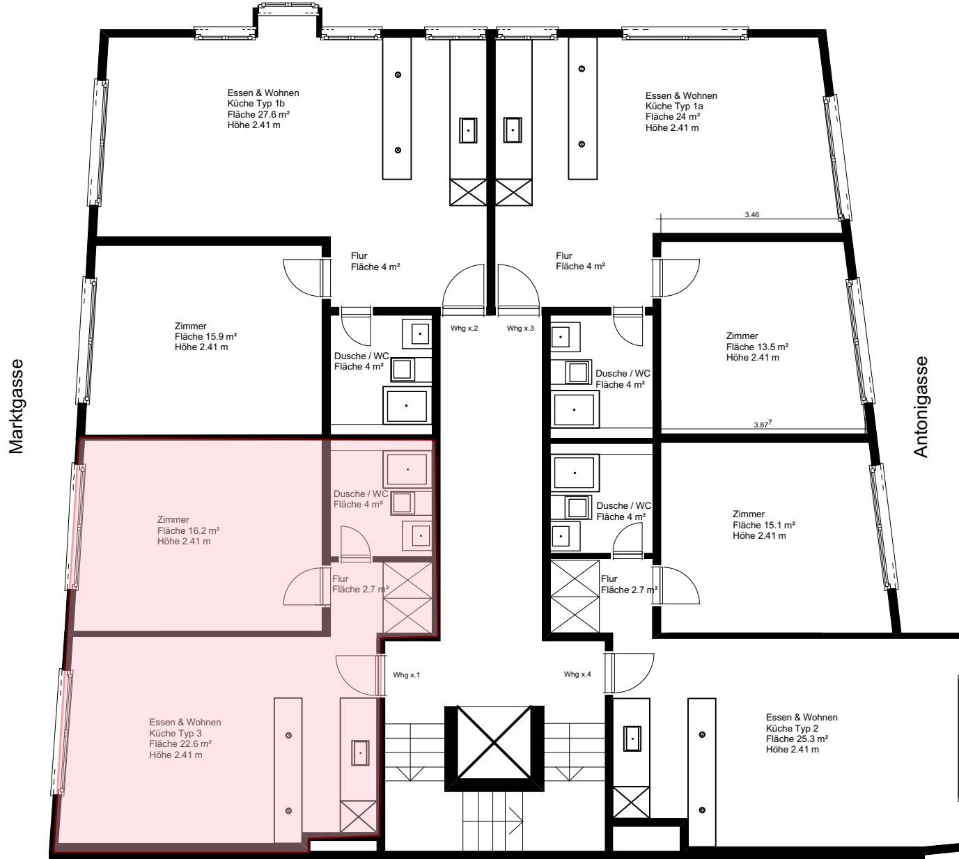
Grundriss 1.OG -4.OG
