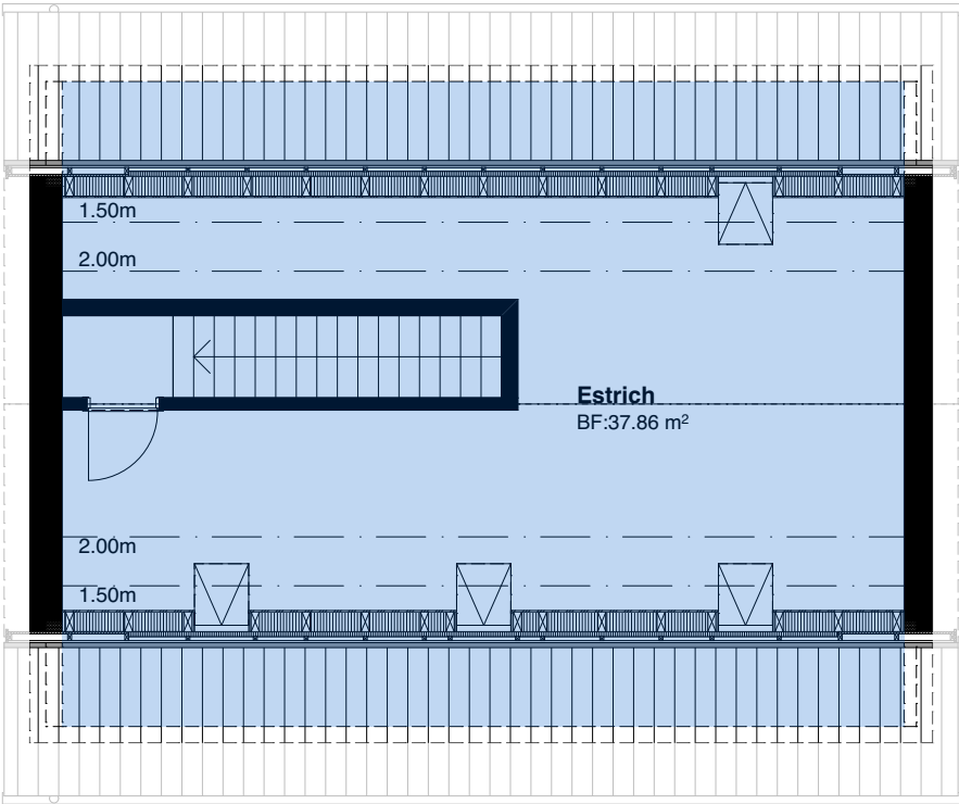
Dachgeschoss EFH
